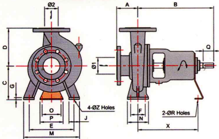
Flanges Dimensions (JIS10K RF)
