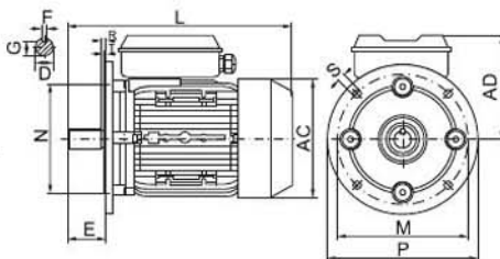
IMB5
