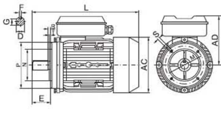
IMB14
