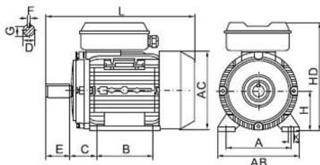
IMB3
